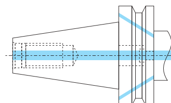
Forma AD+B Refrigeração Central + Flange
