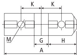
6" a 12" Diâmetro
