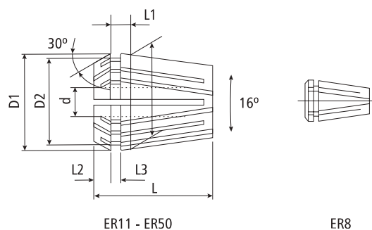
ER11 - ER50
