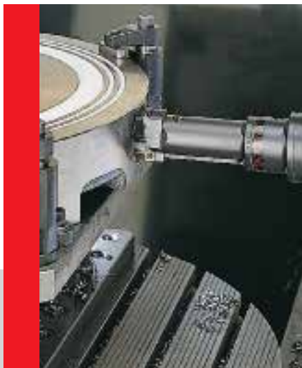
Fig. 1 – Com duas cápsulas SSCC alinhados e no mesmo diâmetro, para operações de desbaste com alta taxa de avanço.
