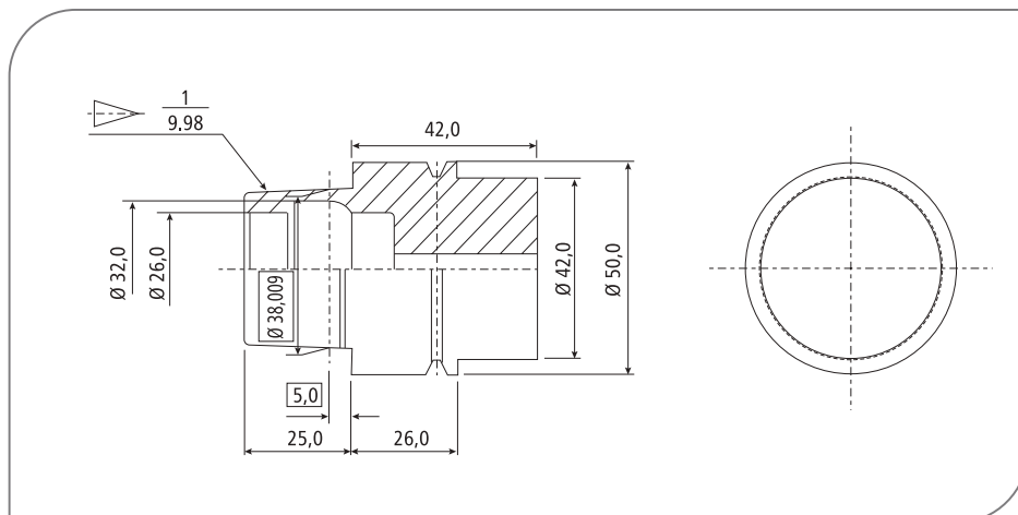
HSK - E50
