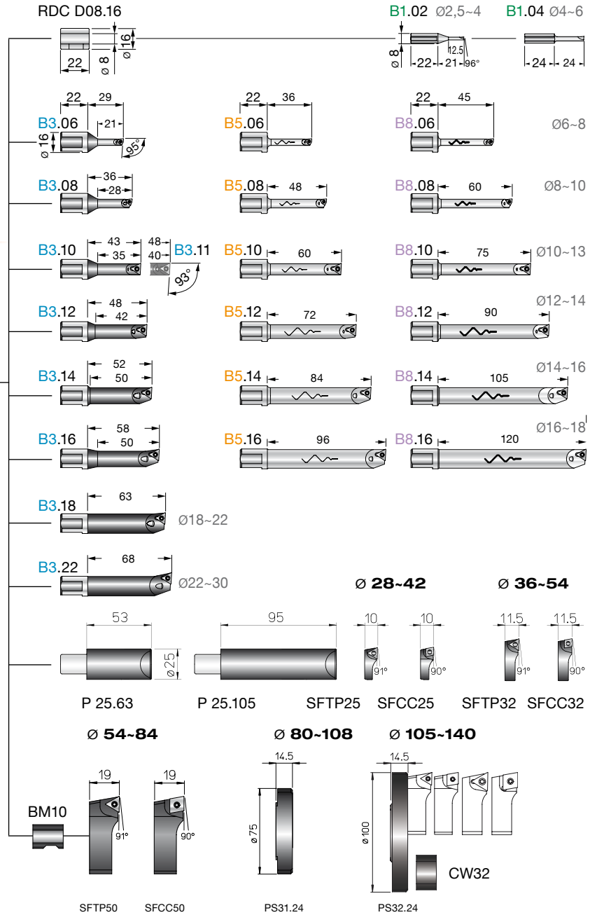
TRM 50 Ø 2.5-140
