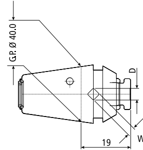
Modelo ERT 40 EXPANSÃO 12 mm
