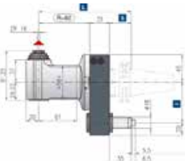
231 T90cn-2,5
