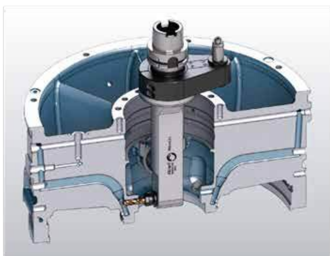
Cabeçote 90° longo
