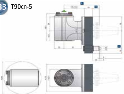
234 TCUn-1,5
