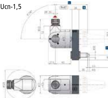
235 TCUn-2,5
