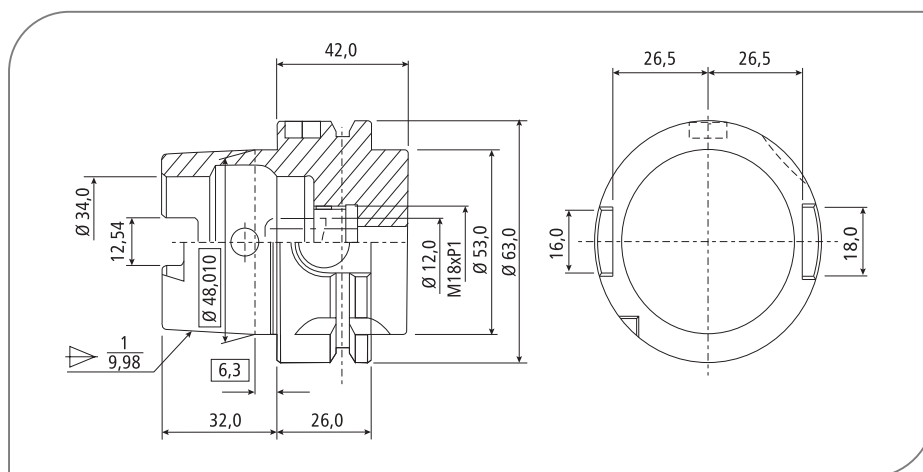
HSK - A63
