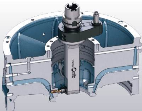
Cabeçote 90° longo
