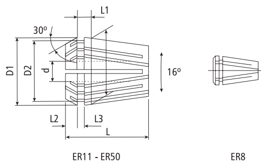
ER11 - ER50
