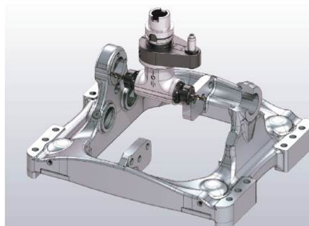
Cabeçote 90° com mandris opostos
