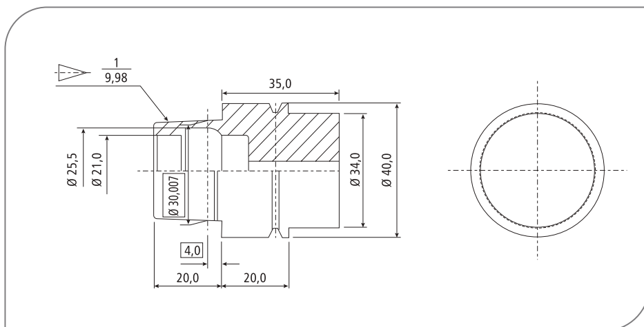
HSK - E40
