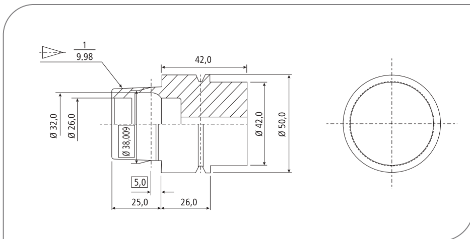
HSK - E50
