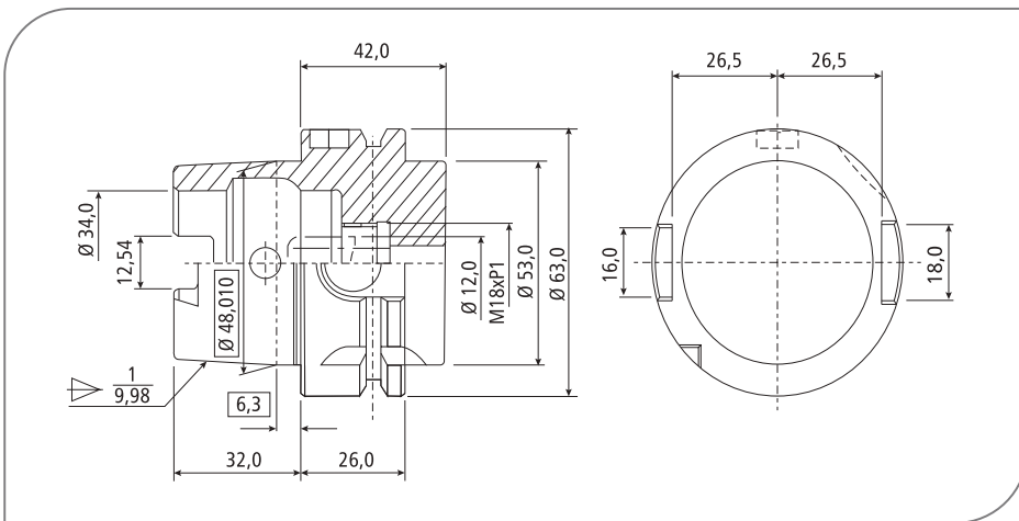
HSK - A63
