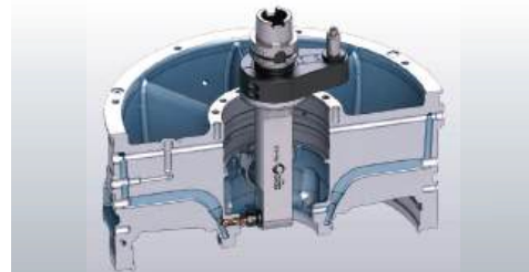
CABEÇOTE 90° LONGO
