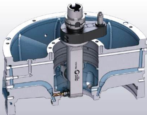
Cabeçote 90° longo
