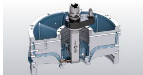
CABEÇOTE 90° LONGO
