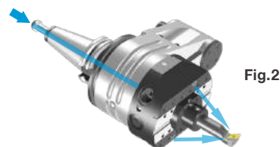
Refrigeração Interna Fig.2
