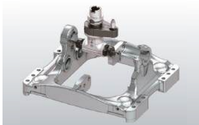
CABEÇOTE FIXO COM MANDRIS OPOSTOS
