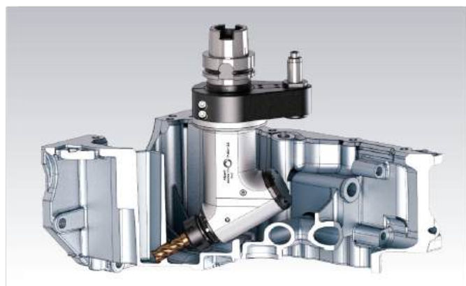
Cabeçote fixo com ângulo variável
