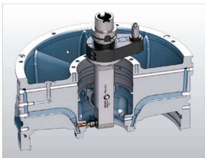
Cabeçote 90° longo
