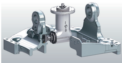
O cabeçote 90° com ou sem flange para grandes peças.
