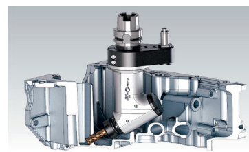
Cabeçote fixo com ângulo variável
