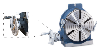
MESA DIVISORA VERTICAL/HORIZONTAL Modelo: HHV-200, 250, 300 e acessórios conforme catálogo
