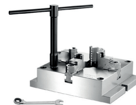
PLACA PARA CENTRO DE USINAGEM COM 4 CASTANHAS
