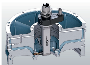
O cabeçote 90° longo
