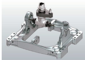
O cabeçote 90° com mandris opostos
