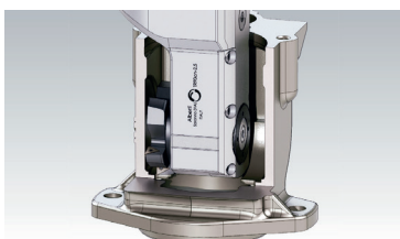
Cabeçote para espaços restritos
