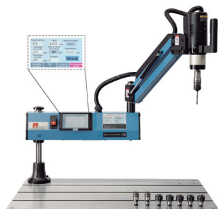
ROSQUEADEIRA ELETRÔNICA COM BRAÇO ARTICULADO Modelo: RE
